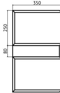
R-18 40x250x350 с фаской А
