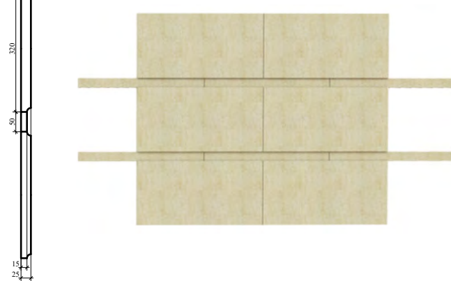
Плитка с фаской В по одной длинной стороне
