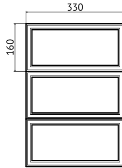
R-06 40x160x330/160 с фаской С
