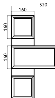
R-16 40x160x160/320 с фаской C
