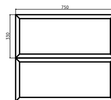
R-08 50x330x750 с фаской А
