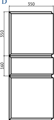
R-13 40x350/160x350 с фаской D
