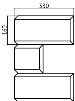
R-07 40x160x330/160 с фаской А
