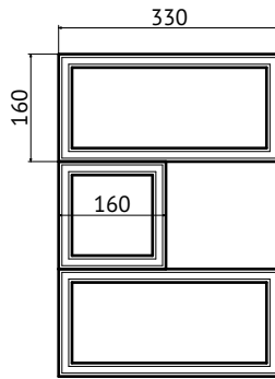
R-08 50x330x750 с фаской А
