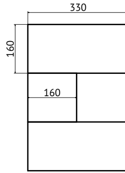
R-04 40x160x330 с фаской С
