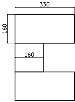
R-03 40x160x330 с фаской В
