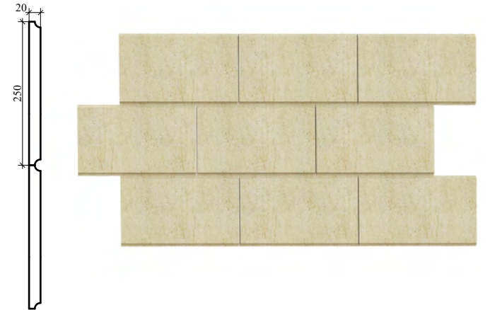
Плитка без фаски со вставкой
