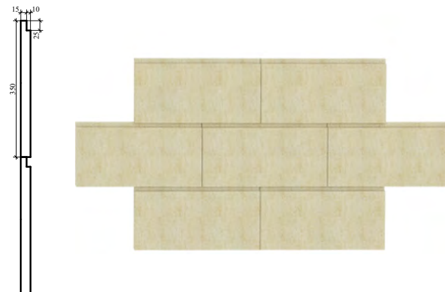
Плитка с фаской В по одной длинной стороне
