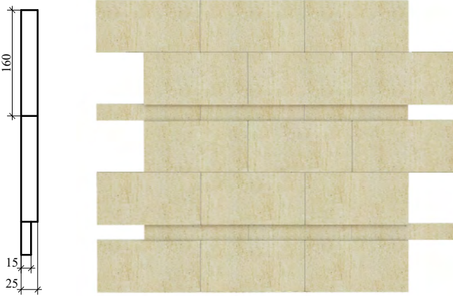
Плитка с фаской D по 2м длинным сторонам со вставкой
